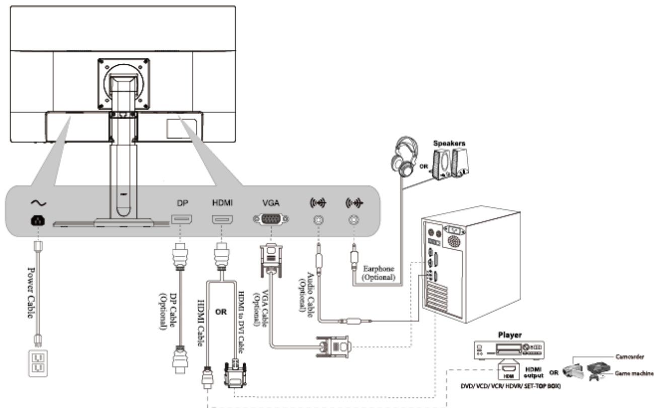
Figura 2. Collegamento al pc
