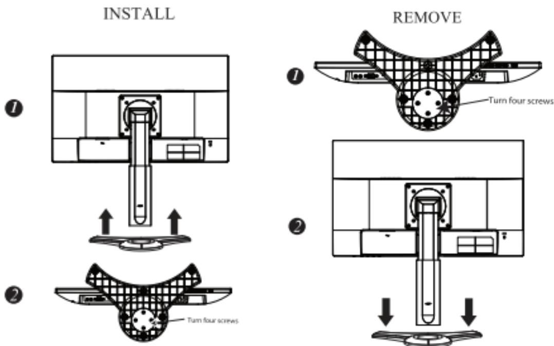
Figura.1. Installazione e Rimozione della Base
